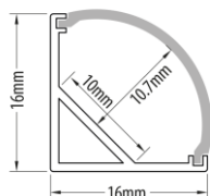
Dimensiones
