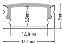
Dimensiones
